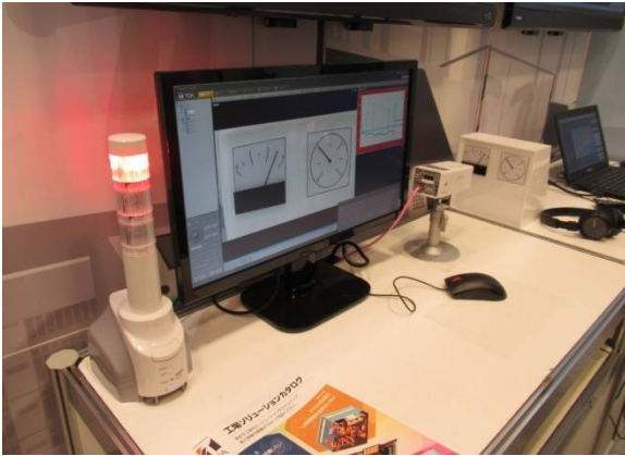
「工場エリア」 計測器をカメラ監視して異常時に警報とランプ点灯
