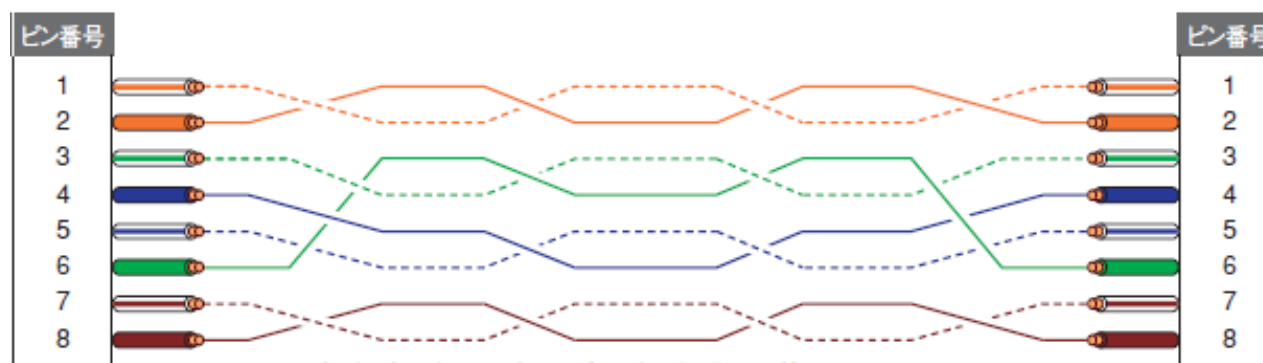
ストレートケーブル結線図 (T568B) 日本国内で標準的に使用されているピンアサインです。
