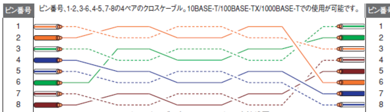
クロスケーブル (568B 4ペアクロス) 結線図
